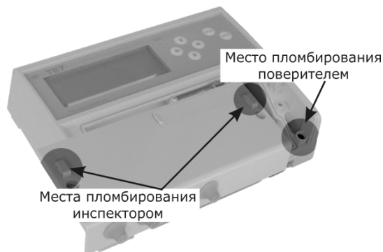
Рис. 1.2 – Места пломбирования вычислителя
