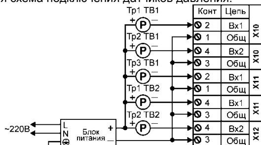
Рис. 4.4 – Пример подключения датчиков давления
