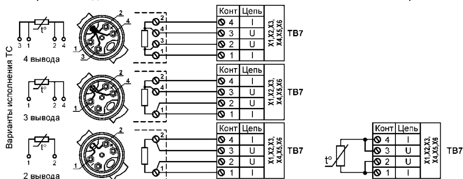
Рис. 4.2 - Варианты подключения ТС
