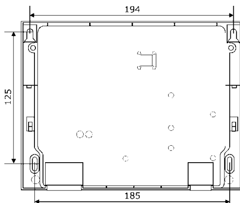
Рис. 4.1 – Схема крепления корпуса ТВ7
