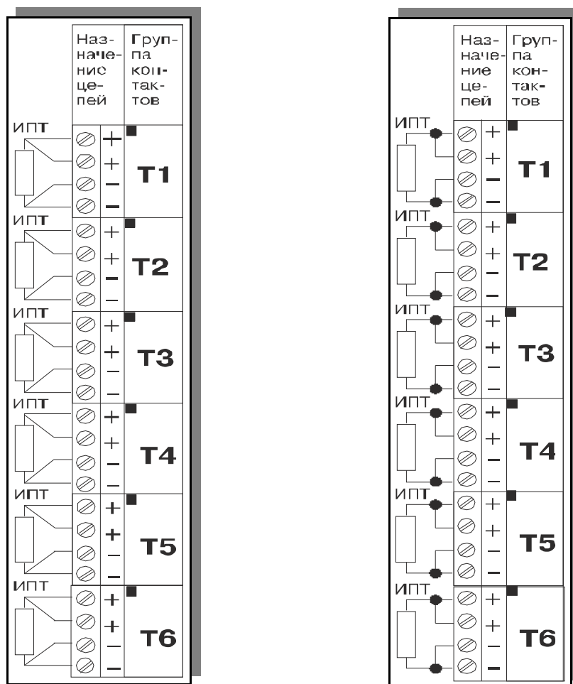
Рисунок Б.2 — Схемы подключения ИПТ к вычислителю по 4-х и 2-х проводным схемам.
