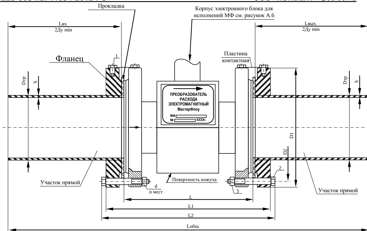
Рисунок А.2а – Поставка фланцевых преобразователей исполнения МФ-5.2Х.Х, МФ-6.2Х.Х, МФ-7.2Х.Х, с комплектом монтажных частей КМЧ МФ №4 с прямыми участками трубопроводов
