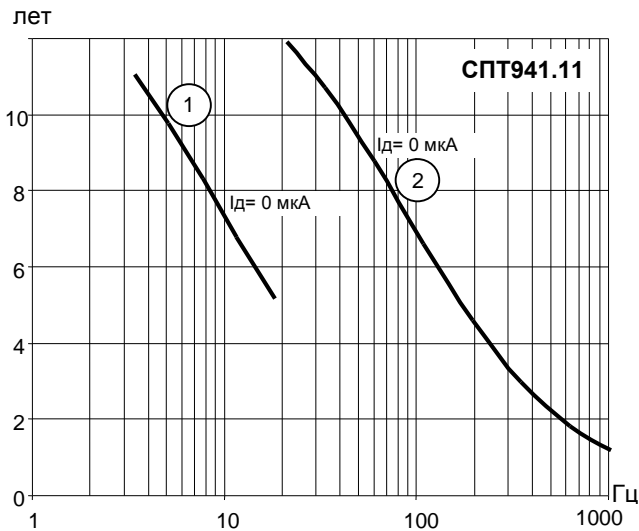
Рисунок 2.1 – Зависимость ресурса батареи (лет) от частоты входных импульсов (Гц) и суммарного среднего тока потребления преобразователей объема I_d .
