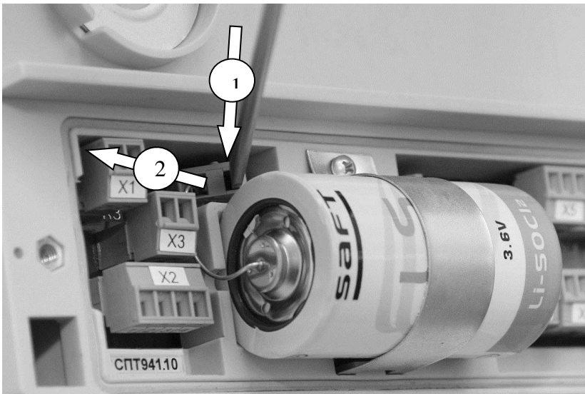
Рисунок 10.2 – Операции при смене батареи. 1 – вставить отвертку в паз и ослабить крепление зажима вывода батареи; 2 – вынуть вывод батареи.
