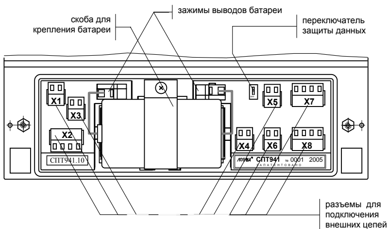
Рисунок 3.2 – Монтажный отсек тепловычислителя СПТ941.10
