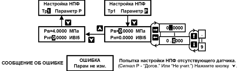
Рисунок 6.2 – Последовательность действий по настройке НФП датчиков давления
