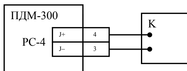
Рисунок 6.3 - Схема подключения средств поверки при проведении поверки измерения силы тока. К – калибратор тока.
